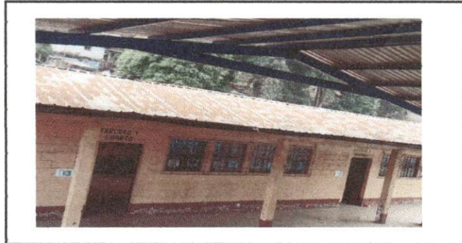
Foto 6: Instalación de bajadas de agua de metal
